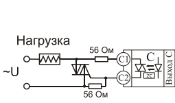
Подключение внешнего симистора
