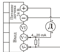
датчик с унифицированным токовым сигналом и внешним питанием 24 В
