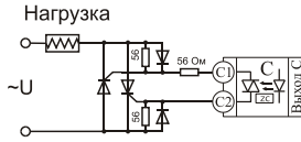
Подключение внешних тиристоров
